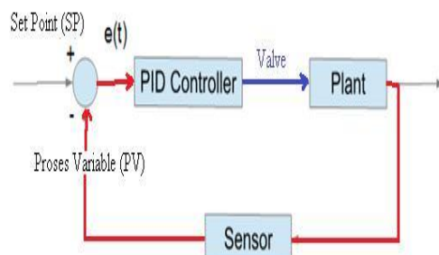
Gambar 12. Blok Diagram PID Sistem Siklus Tertutup
