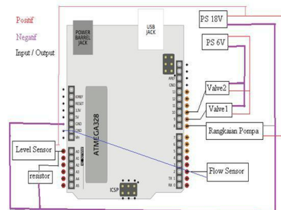
Gambar 7. Rangkaian Arduino.
