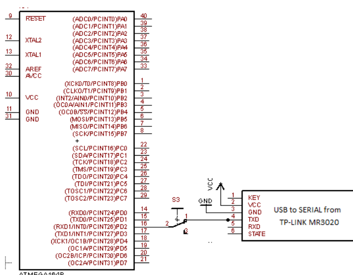
Gambar 9. Rangkaian TP-LINK MR3020 pada ATMEGA164p
