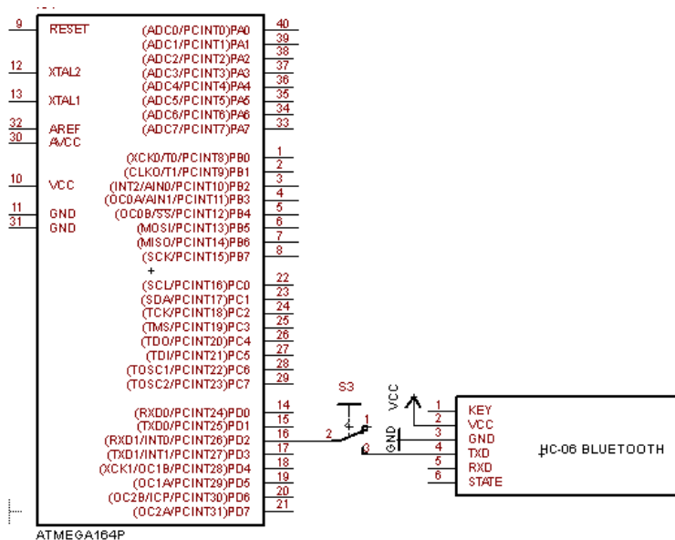
Gambar 7. Rangkaian Bluetooth HC-06 pada ATMEGA164p
