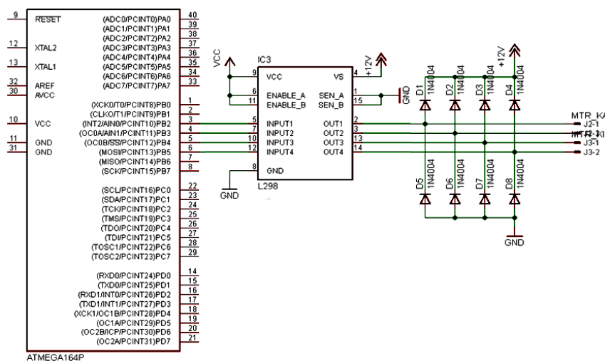
Gambar 5. Skematik Rangkaian Driver Motor Menggunakan L298N
