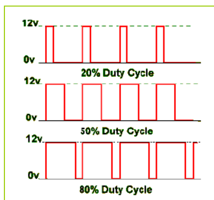
Gambar 1. Ilustrasi persentasi PWM
