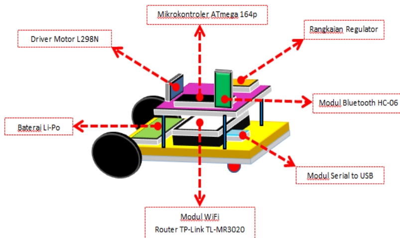
Gambar 4. Skematik Sistem Minimum Mikrokontroler ATMEGA164p
