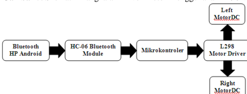
Gambar 5. Skematik Rangkaian Driver Motor Menggunakan L298N
