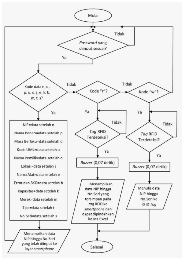
Gambar 3. Diagram Alir Perancangan Sistem
