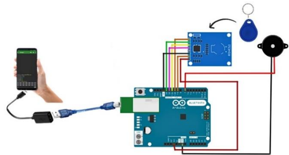
Gambar 4. Skematik Rangkaian Elektronika
