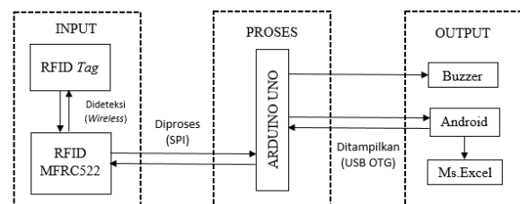
Gambar 2. Diagram Blok Kerja Sistem
