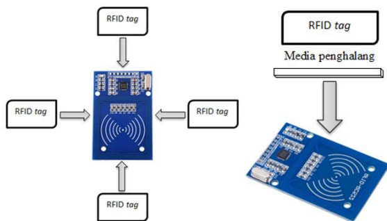
Gambar 5. Posisi tag dengan dan/atau tanpa media penghalang
