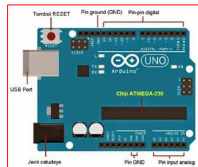
Gambar 1. Arduino UNO
