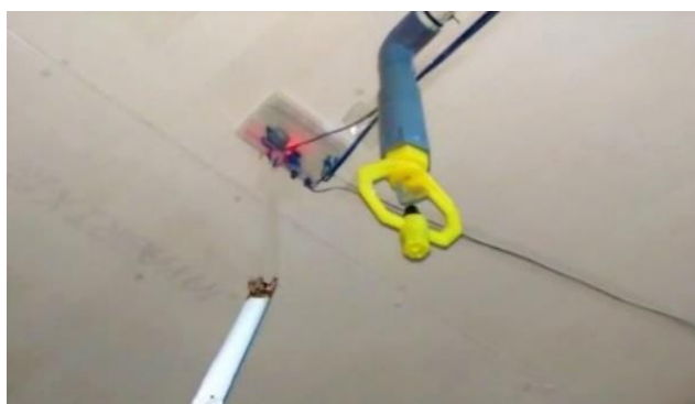
Gambar 4. Pengujian Sensor MQ7
