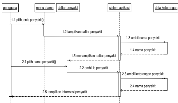
Gambar 3. Sequence Diagram untuk Menu Deteksi Penyakit
