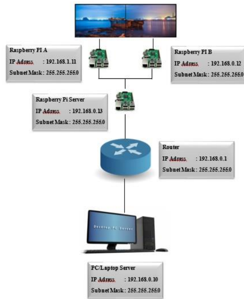
Gambar 3. Topologi Logik
