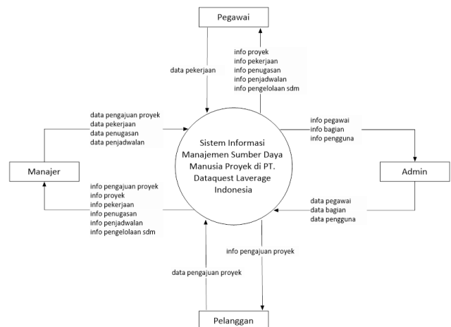
Gambar 22 Diagram Konteks
