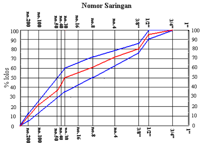
Gambar 1 Kurva gradasi Lataston HRS-WC
