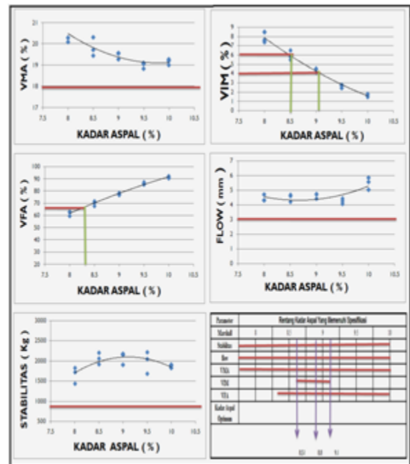
Gambar 4. Penentuan KAO untuk filler dari 50% No.200 + 50% Spent Catalyst
