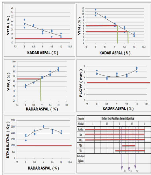
Gambar 5. Penentuan KAO untuk 100% filler Spent Catalyst
