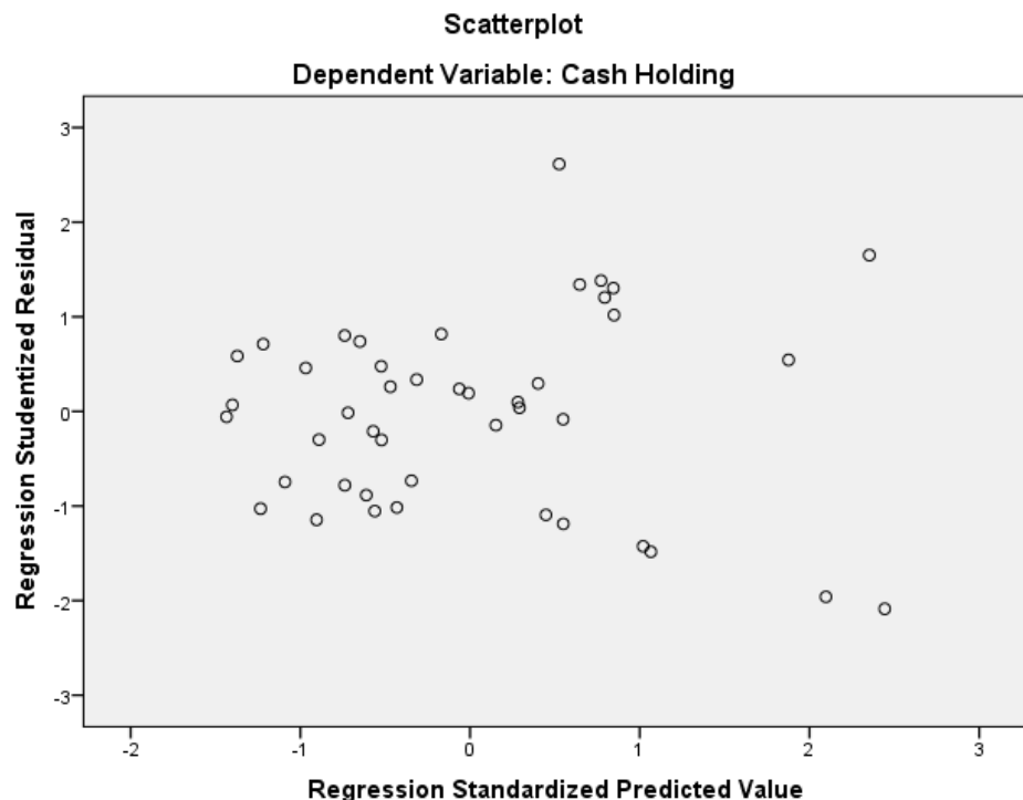
Gambar 4.1 Uji Heteroskedastisitas
