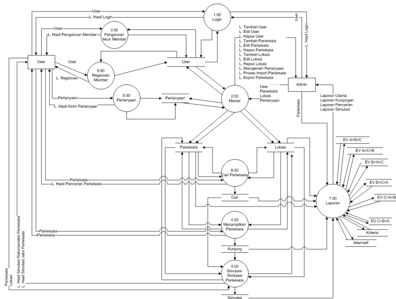
Gambar 4.3 DFD Level 1 Sistem Informasi Pendukung Keputusan Pariwisata Berbasis Web
