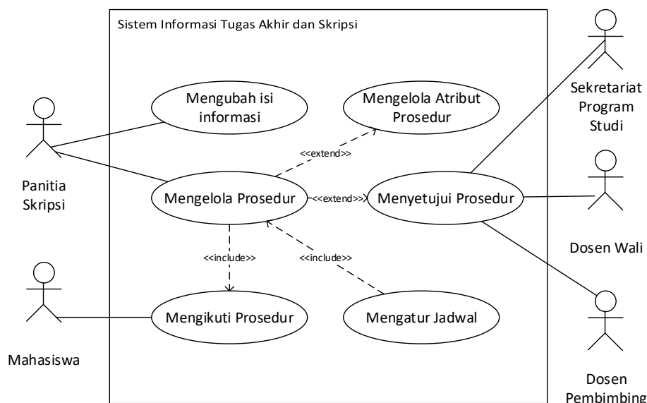
Gambar 3. Use Case Sistem yang Diusulkan
