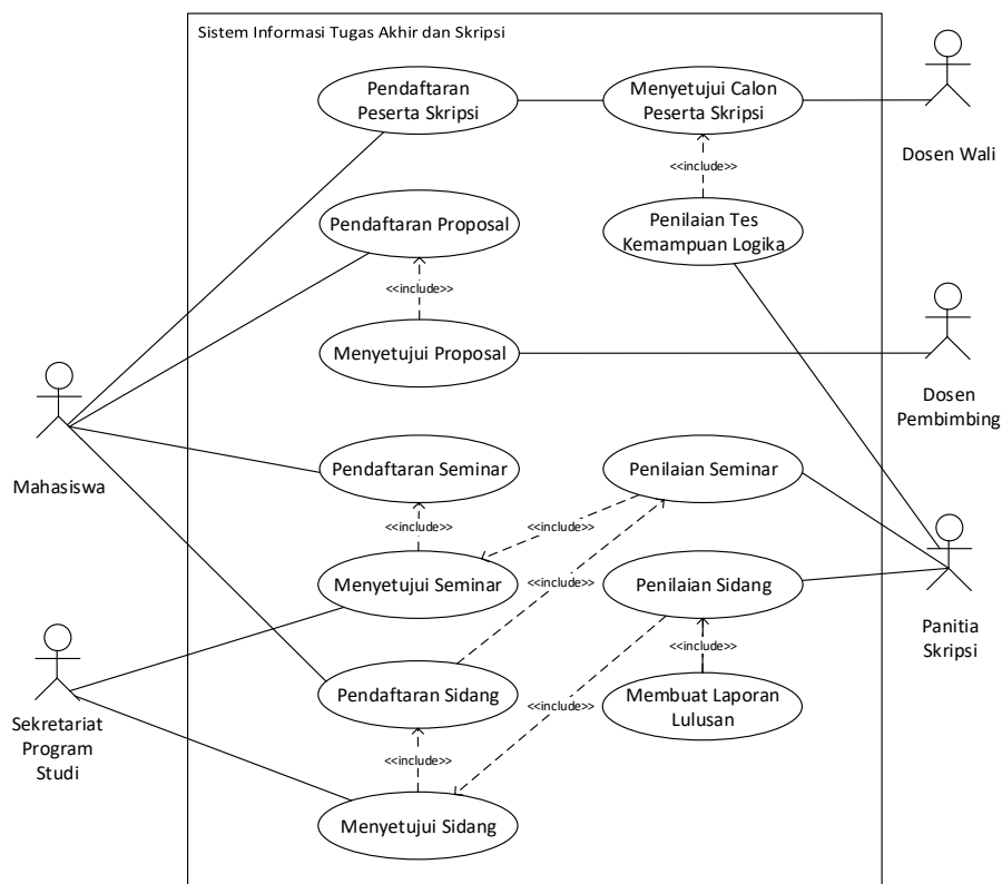
Gambar 2. Use Case sistem yang sedang berjalan
