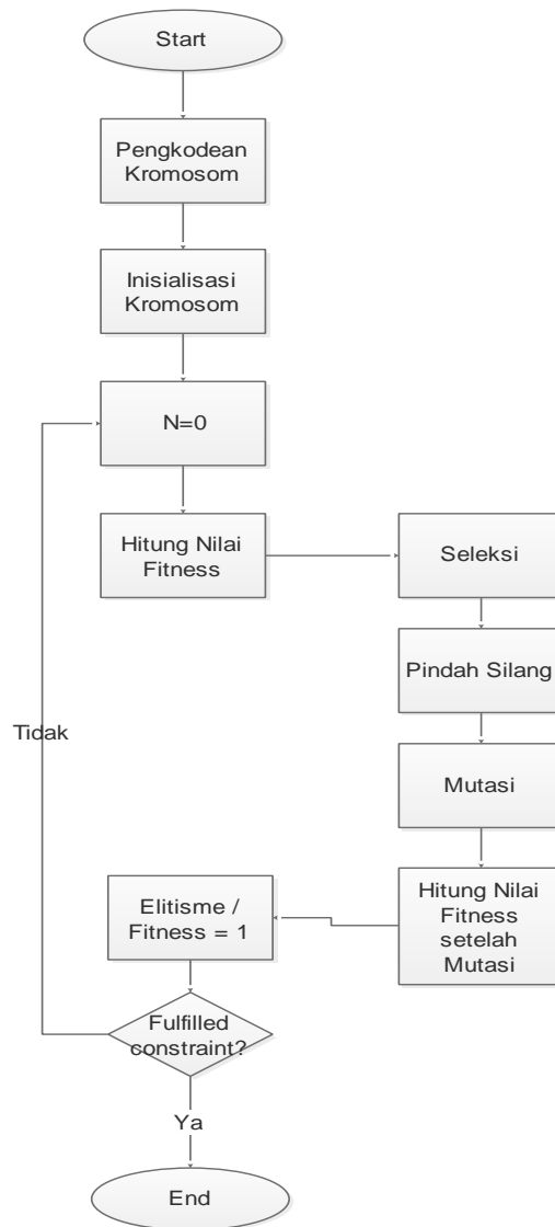
Gambar 4 Alur Algoritma
