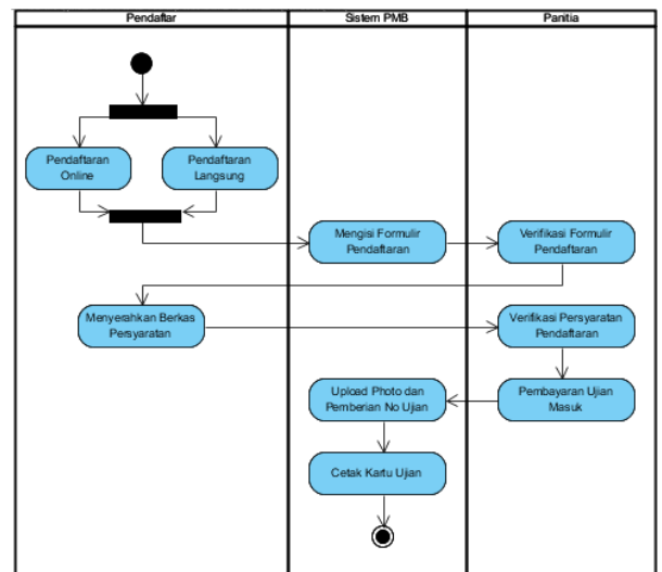
Gambar 2. Activity Diagram Sistem PMB yang berjalan
