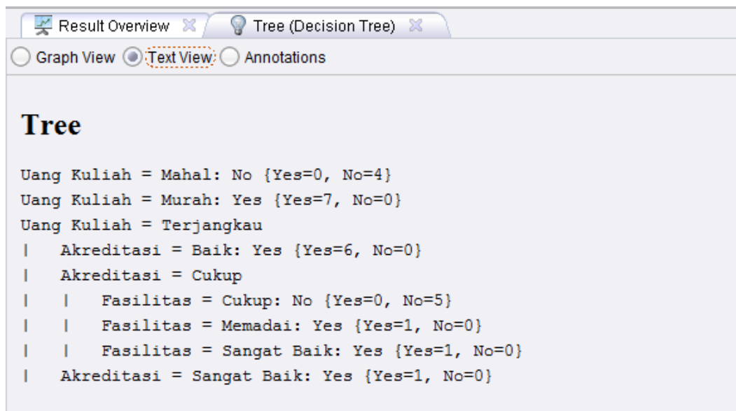
Gambar 8. Hasil Keputusan Pengujian Berdasarkan Software RapidMiner
