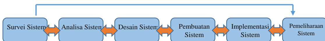
Gambar 2. Tahap Pengembangan Sistem dengan Model Iterasi
