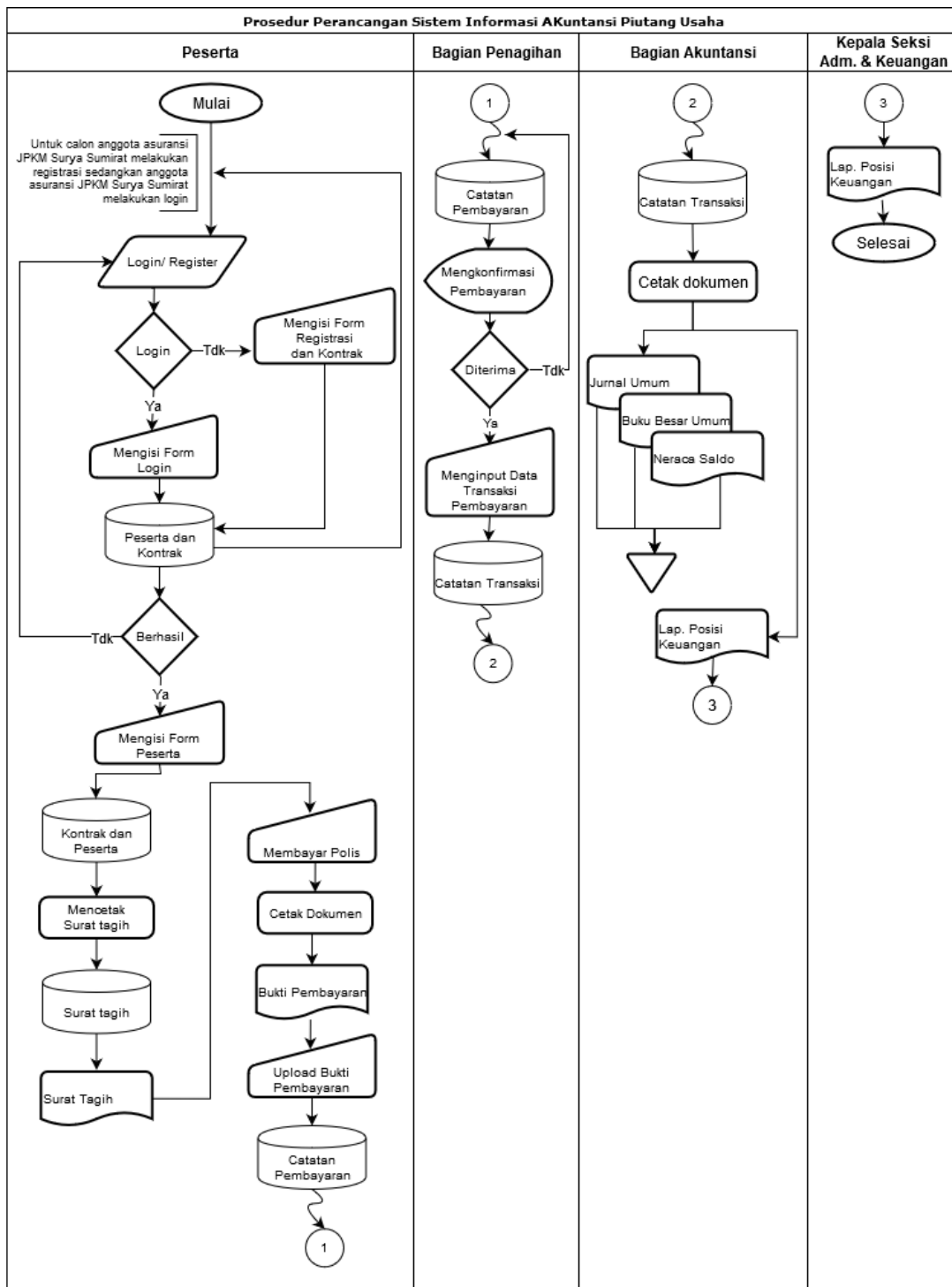
Gambar 4. Bagan Alir Sistem yang Diusulkan
