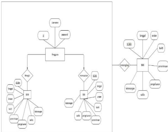
Gambar 8 ERD
