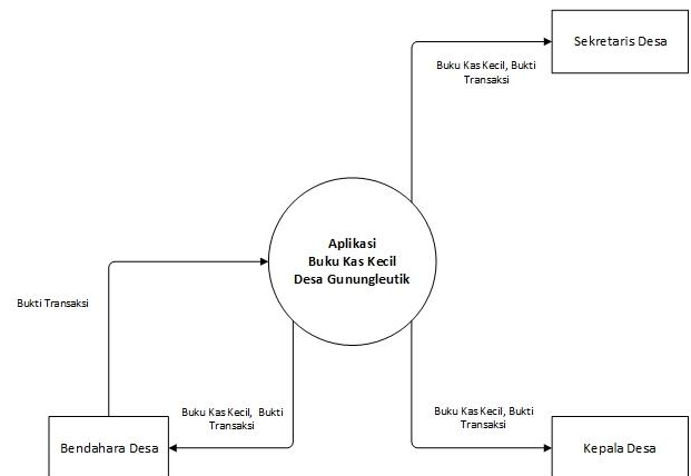
Gambar 6 Diagram Konteks
